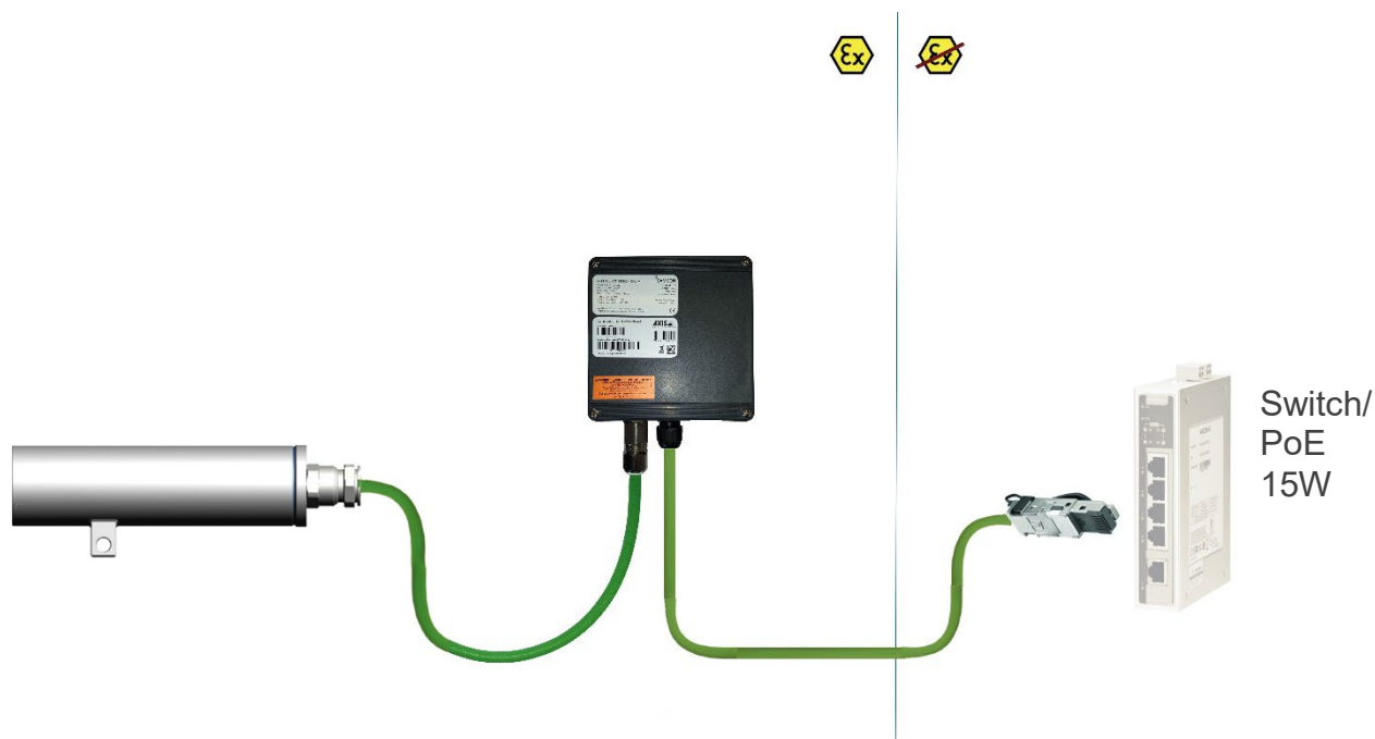
Bild 5-8 ExTB-3 -> Sicherer Bereich
