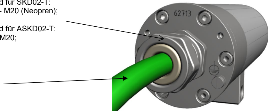
Bild 5-2 Ex-d Kabelverschraubung und Zuleitung
