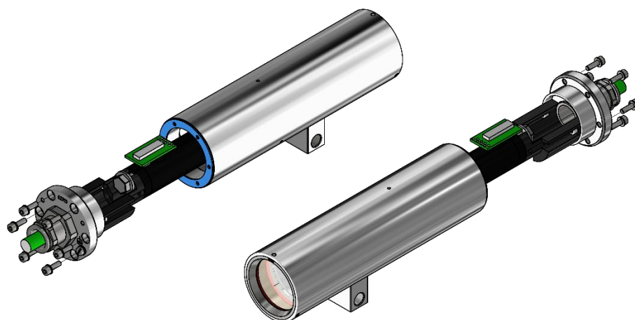
Bild 6-1 Öffnen der ExCam® microTube IP
